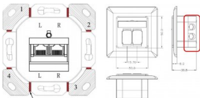
1-4: breakable edges space-saving installation 1-4: abbrechbare Ecken für platzsparende Installation
