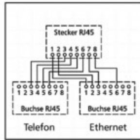
Schaltbild / Wiring diagram
