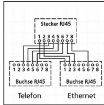
Schaltbild / Wiring diagram
